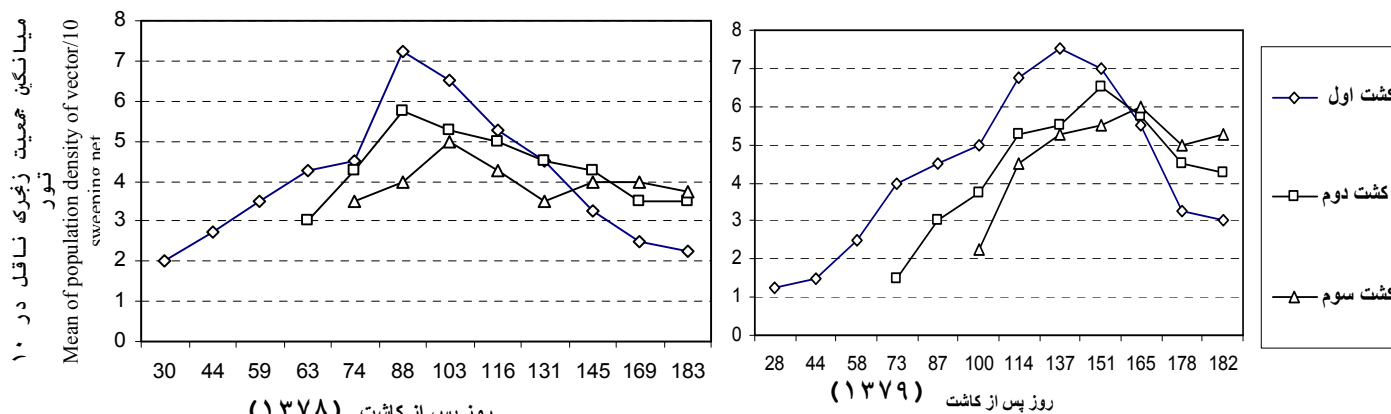
شکل ۱: میانگین جمعیت زنجبرک‌ها در تور ۱۰×۱۰ متر مربعی در روز پس از کاشت (۲۰۰۰) Days after planting (۲۰۰۰) در کاشتهای مورد مطالعه در شهرستان مبارکه طی سالهای ۱۳۷۸ و ۱۳۷۹
